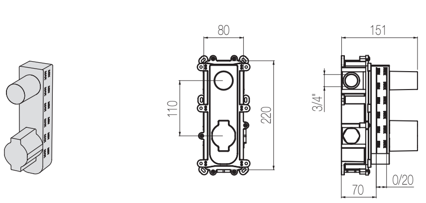
Parte incasso / Built-in part
