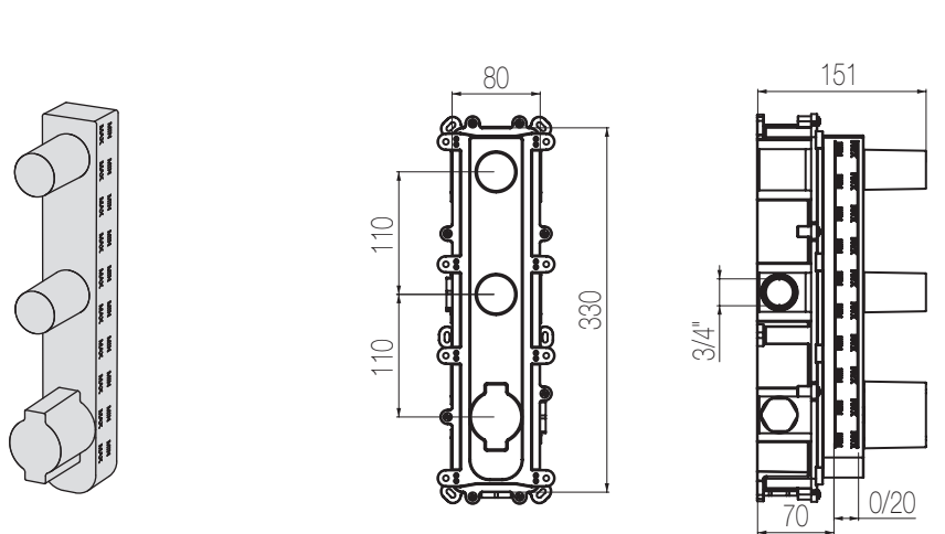
Parte incasso / Built-in part
