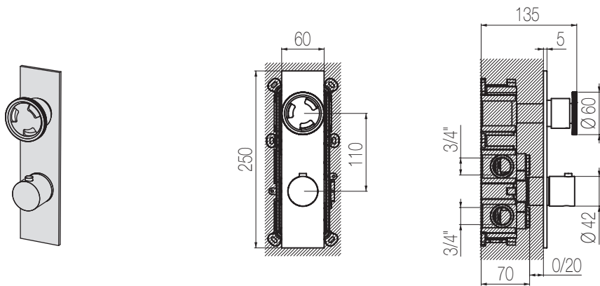
Parte estetica / External part
