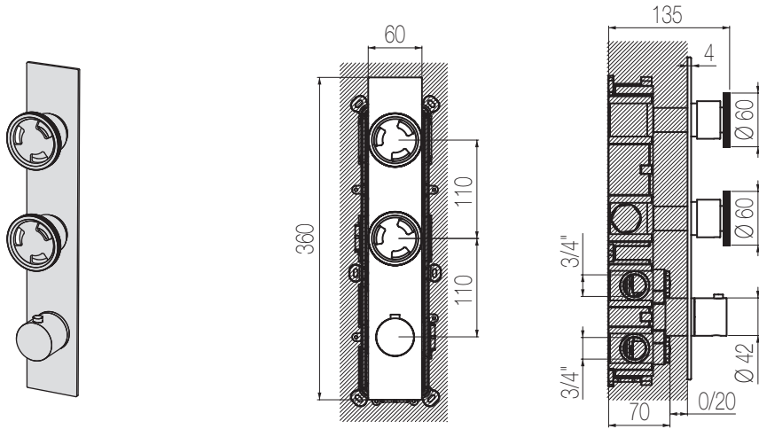
Parte estetica / External part
